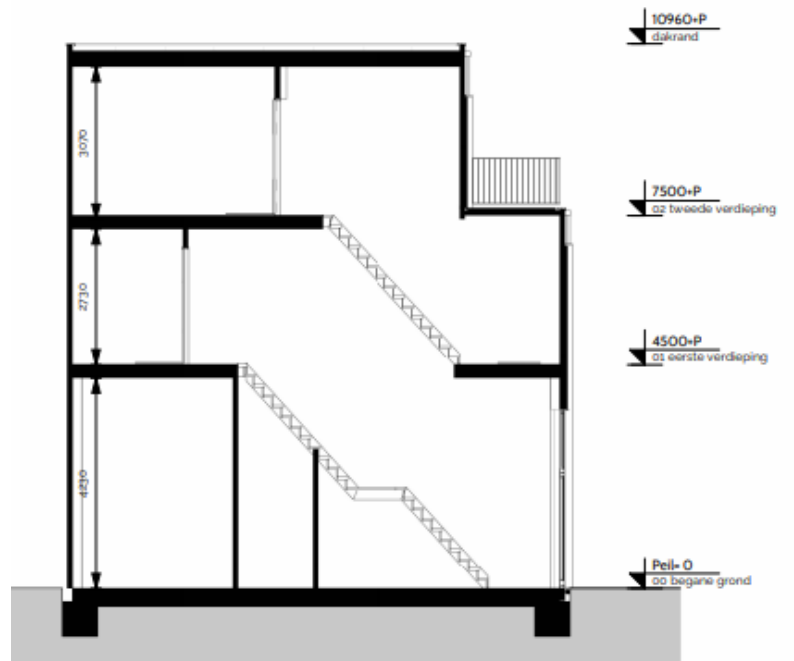
doorsnede
