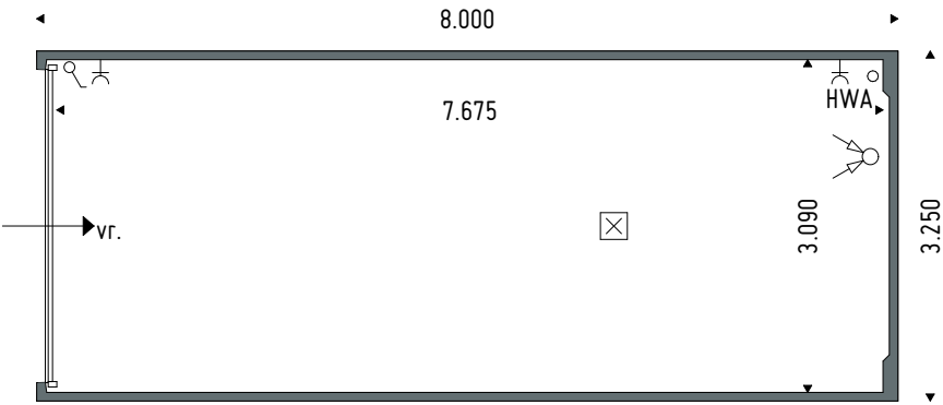
Plattegrond
