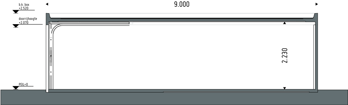
Langsdoorsnede
