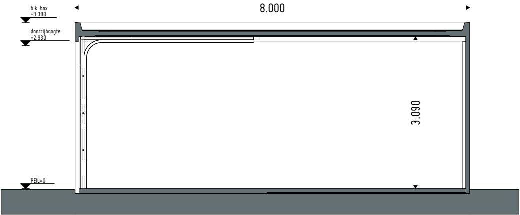
Langsdoorsnede
