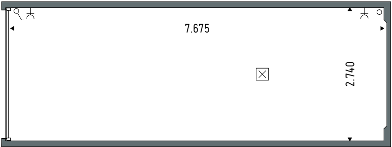
Plattegrond
