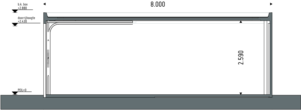
Langsdoorsnede
