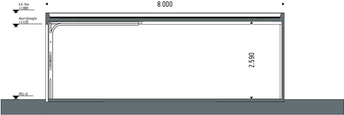
Langsdoorsnede
