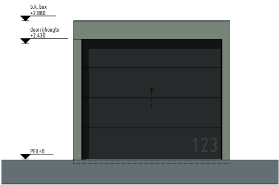
Voorgevel
