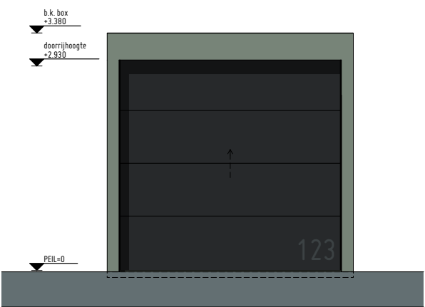
Vorgevel
