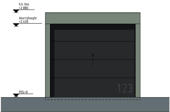
Voorgevel
