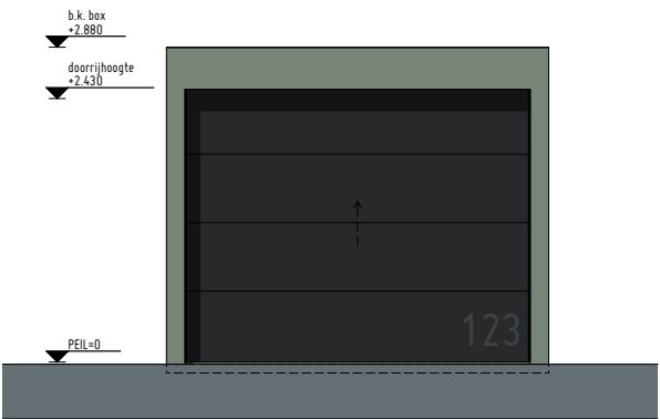
Voorgevel
