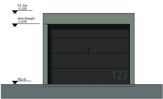
Voorgevel
