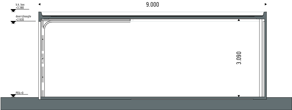
Langsdoorsnede
